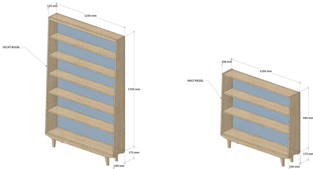
Obr. 10: Axonometria pôvodných drevených regálov na knihy
