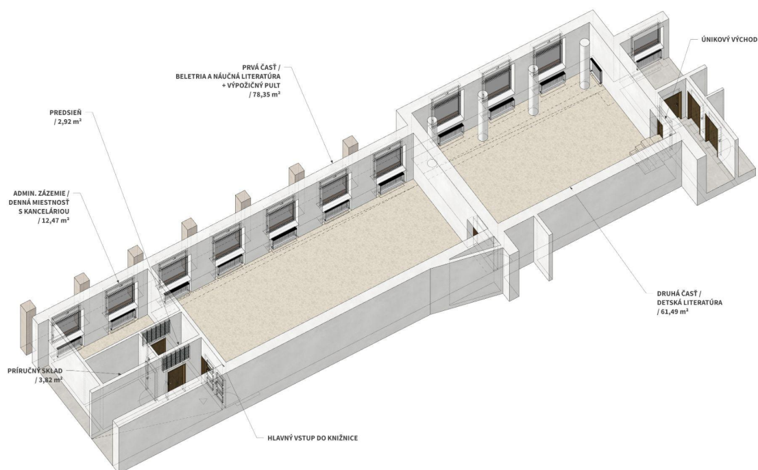
Obr. 5: Axonometria súčasného priestoru knižnice
